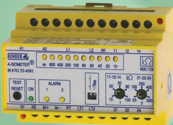
A-ISOMETER® IR470LY2-4061
